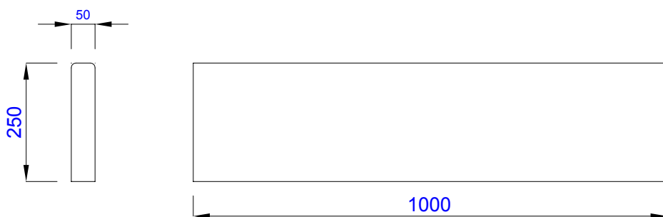
MODULO STANDARD 50 h.250 peso 27 kg.
