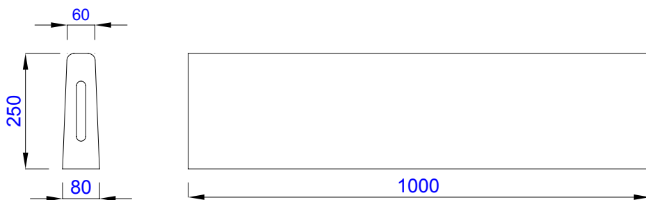
MODULO STANDARD 60x80h.250 peso 40 kg.
