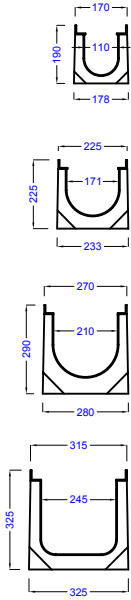
SEZIONE
