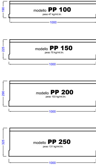
VISTA LATERALE
