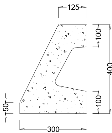
sezione
