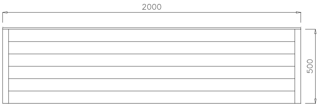
MODELLO industrial (vista davanti) peso 63 kg.
