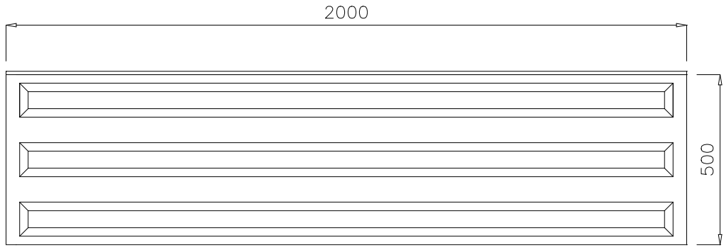
MODELLO industrial (vista dietro) peso 63 kg.
