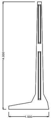
vista frontale
