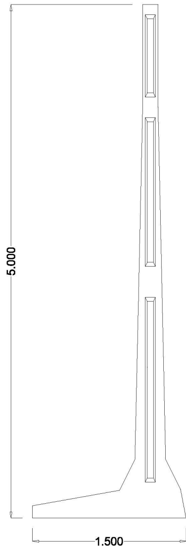
vista frontale
